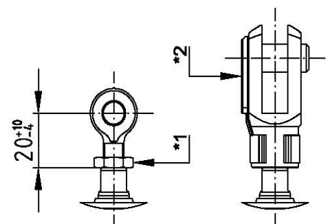
Abbildung 6: Kolbenstangenaufhängung
